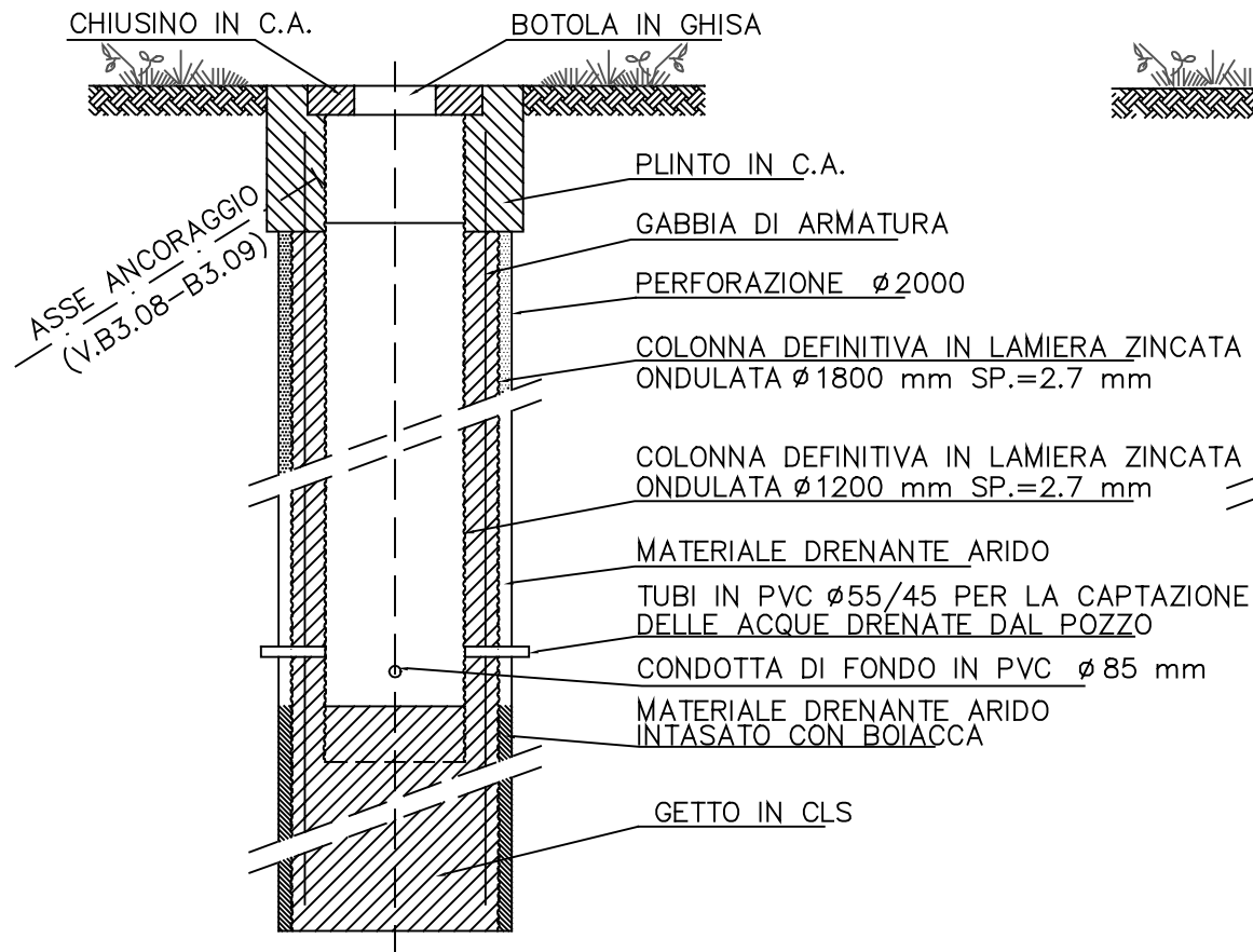
POZZO DRENANTE STRUTTURALE
