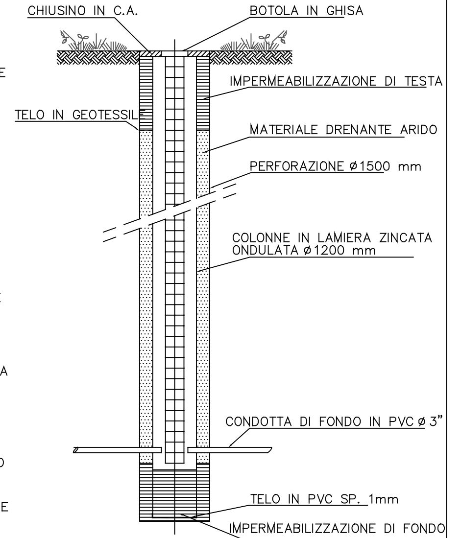
POZZO DRENANTE ISPEZIONABILE
