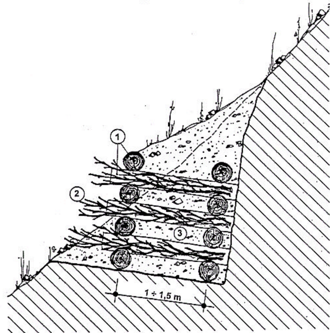
Palificata in legname a due pareti
