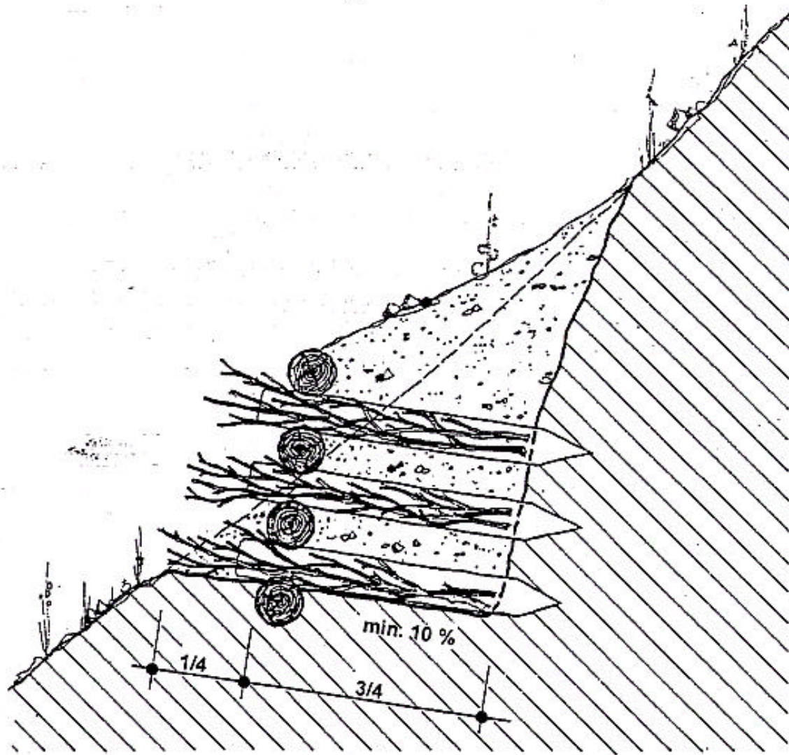
Palificata in legname ad una parete
