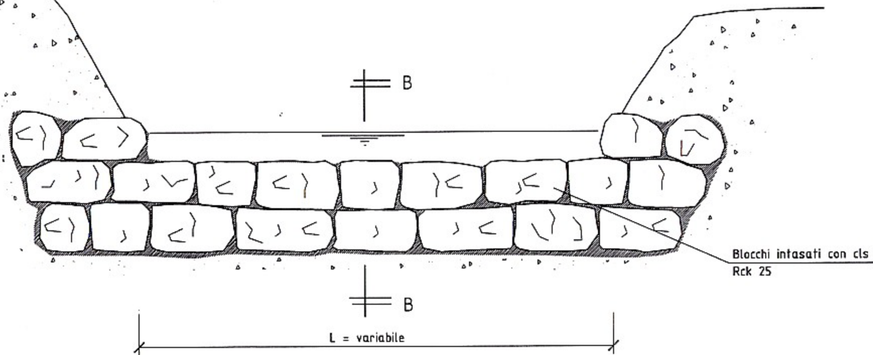
SEZIONE A-A
