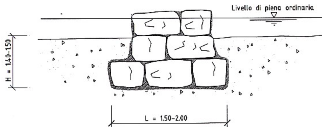
SEZIONE B-B
