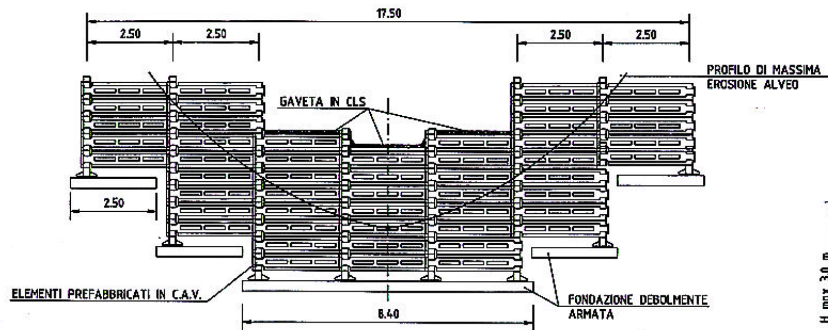
PROSPETTO
