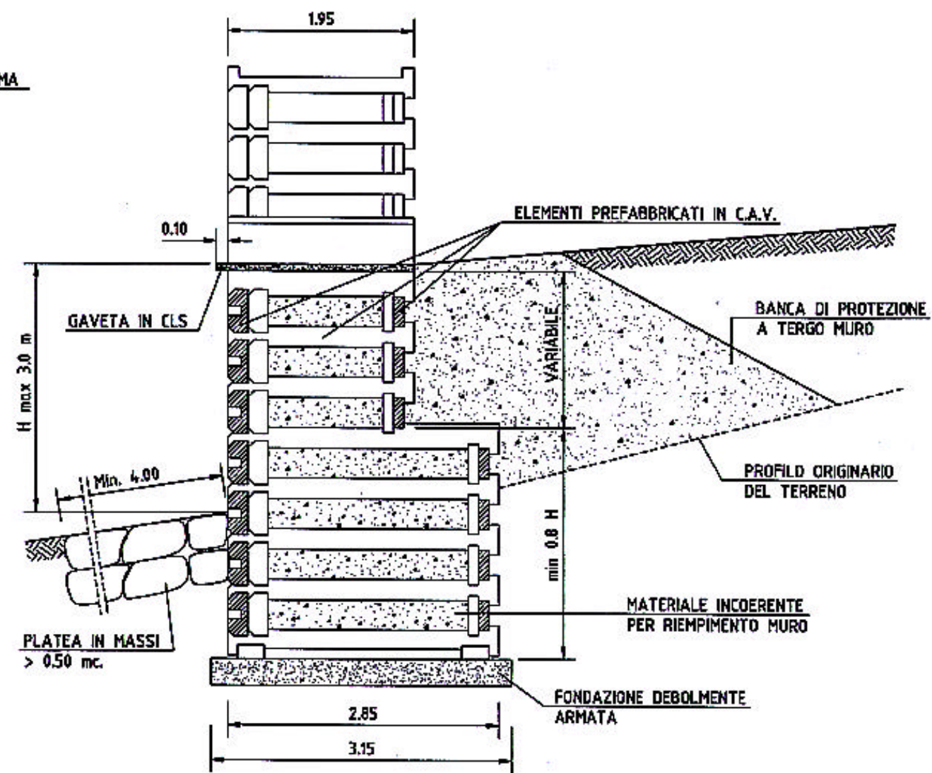
SEZIONE TIPO
