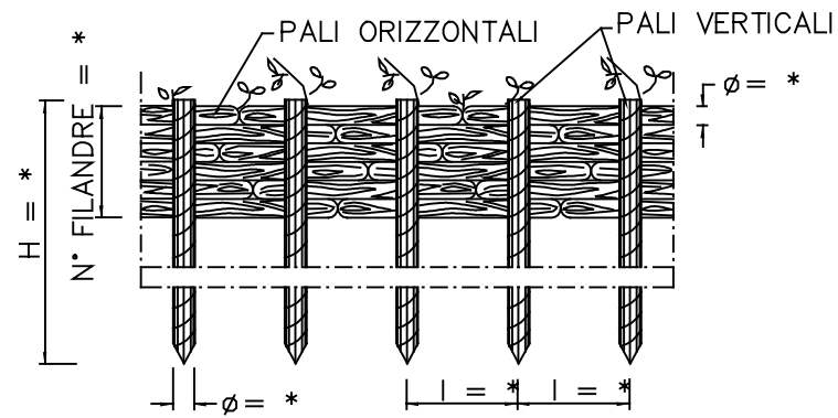
PROSPETTO
