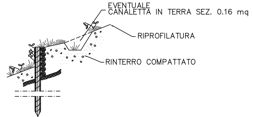
SEZIONE
