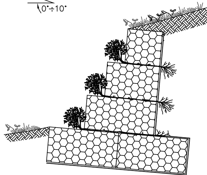
CON TALEE DI SALICE
