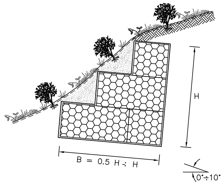
CON CUNEO VERDE ESTERNO
