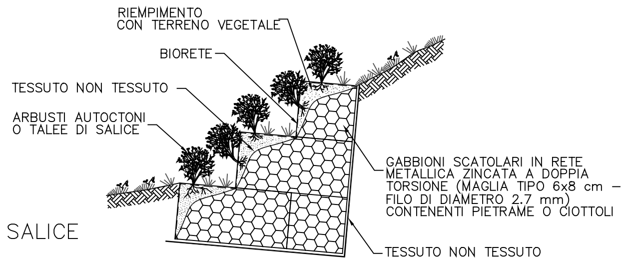
CON CUNEO VERDE INTERNO
