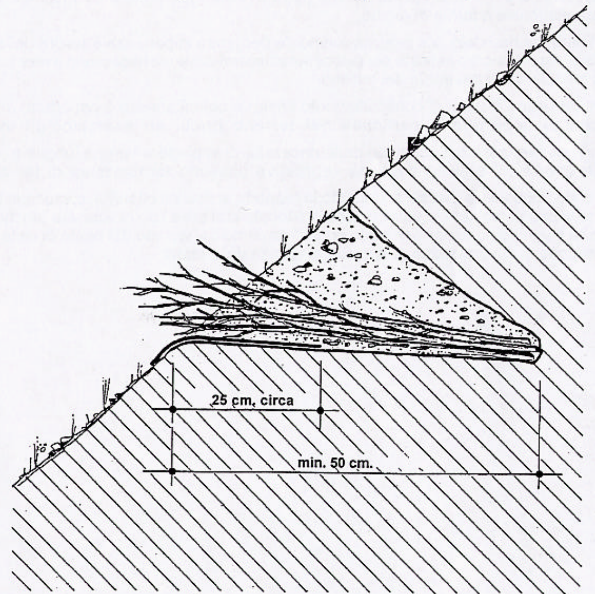
Gradonata con talee (con rinforzo longitudinale)
