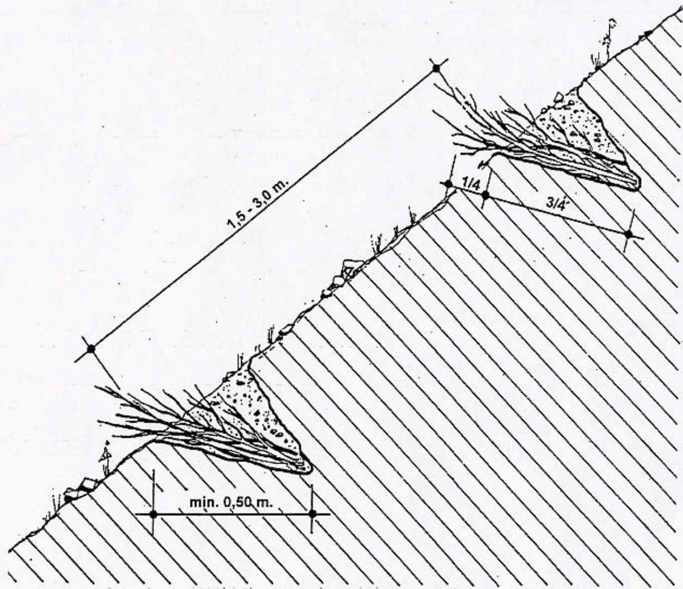
Gradonata con talee
