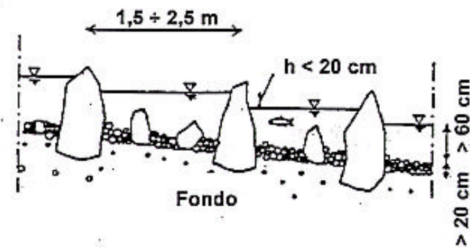
Sezione
