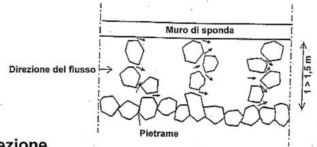
Pianta
