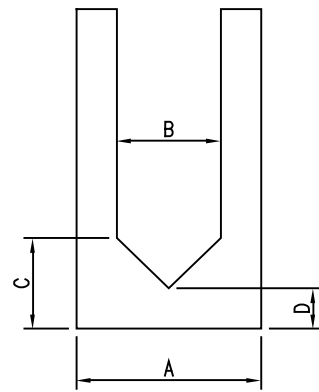
Particolare deflettore
