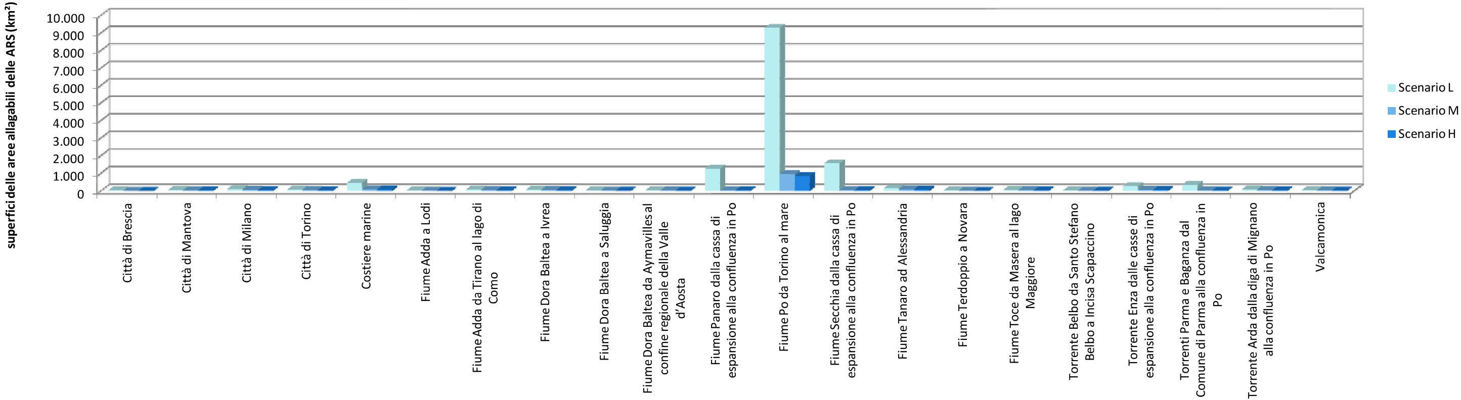
Aree allagabili comprese nelle Aree a Rischio Significativo (ARS)
