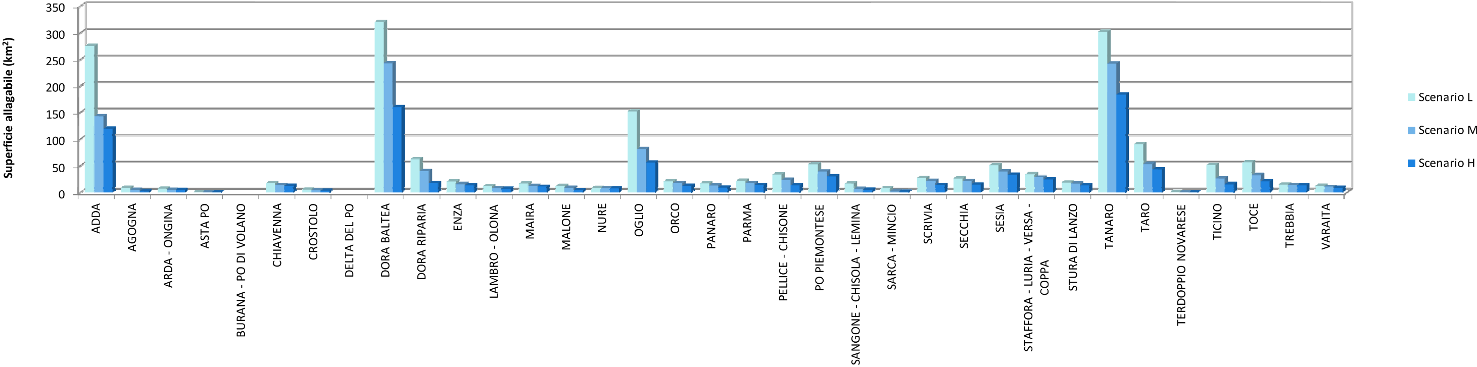
Superficie allagabile per bacino (km 2 ) - Ambito Reticolo Secondario Collinare Montano (RSCM)
