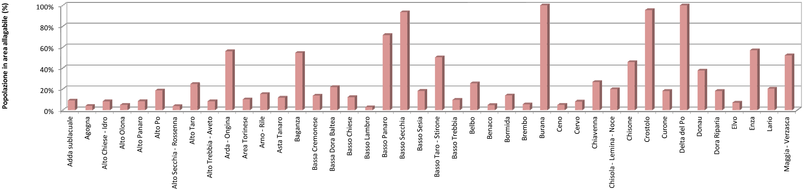
Popolazione potenzialmente esposta alle alluvioni nei sottobacini (%)
