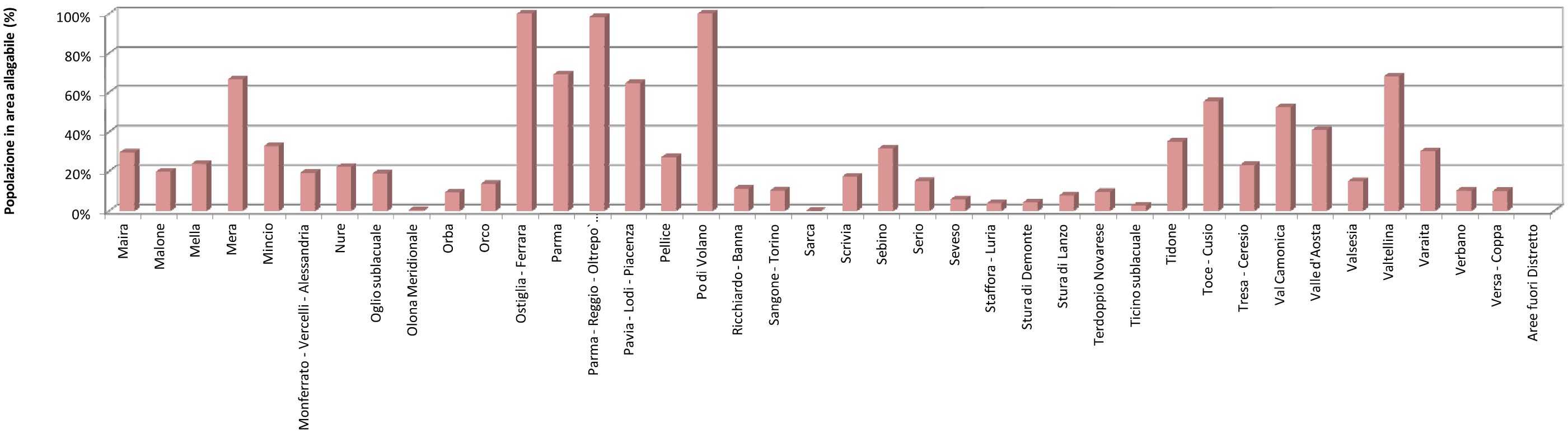
Popolazione potenzialmente esposta alle alluvioni nei sottobacini (%)
