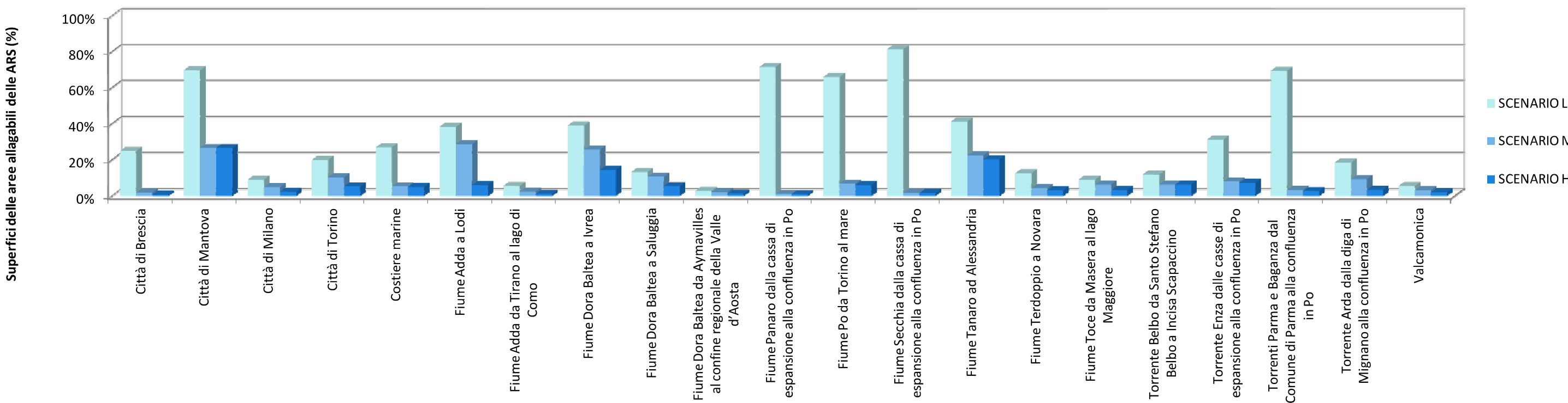
Aree allagabili comprese nelle Aree a Rischio Significativo (ARS)
