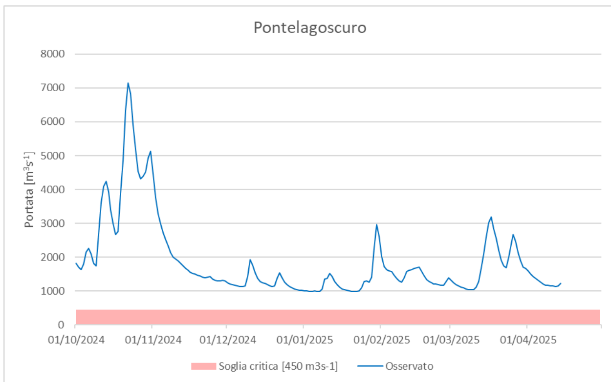
Figura 7: Andamento della portata giornaliera nella sezione idrometrica di Pontelagoscuro al 14 aprile confrontata con la soglia critica per quanto riguarda l'intrusione salina pari a 450 \text{ m}^3\text{s}^{-1} .
