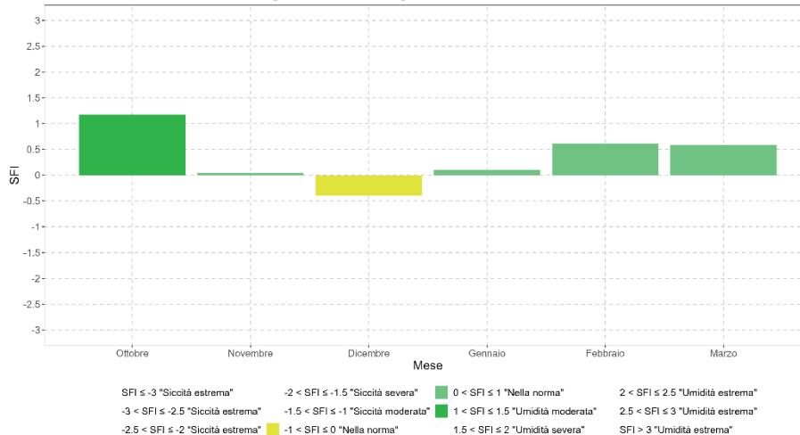
Borgoforte: Anno idrologico Ottobre 2024 - Marzo 2025
