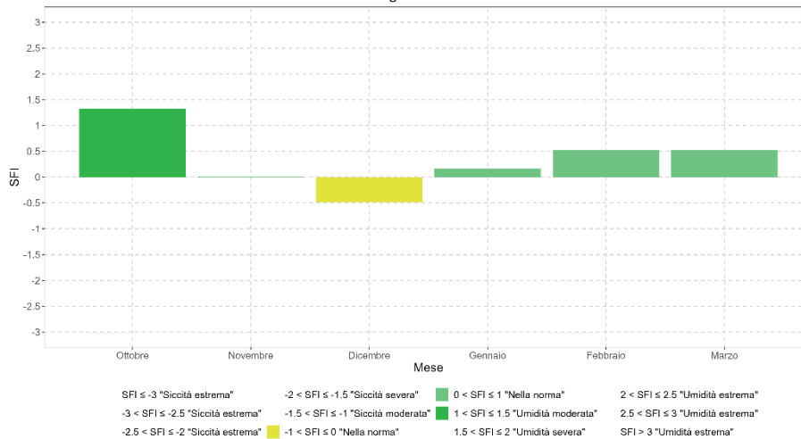
Boretto: Anno idrologico Ottobre 2024 - Marzo 2025
