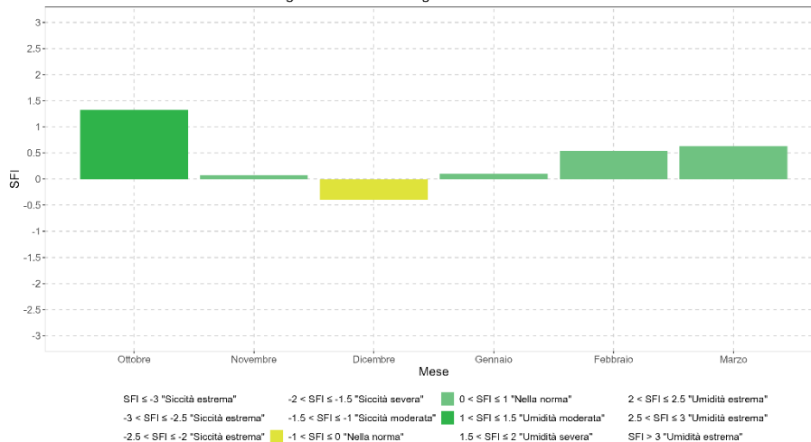
Pontelagoscuro: Anno idrologico Ottobre 2024 - Marzo 2025
