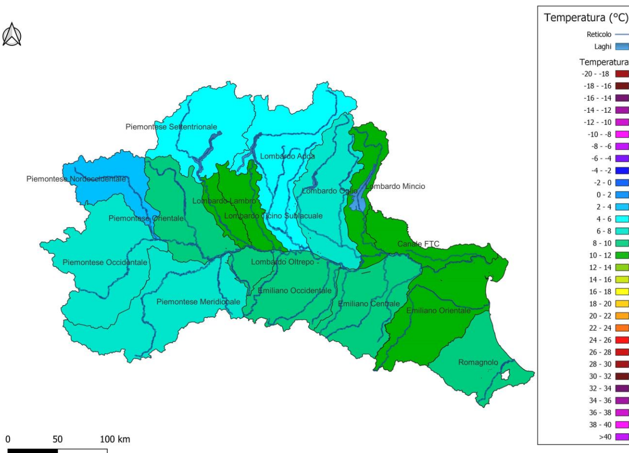
Figura 4: Rappresentazione delle temperature medie mensili nelle aree idrografiche del Distretto. Dati aggiornati al 31 marzo 2025.
