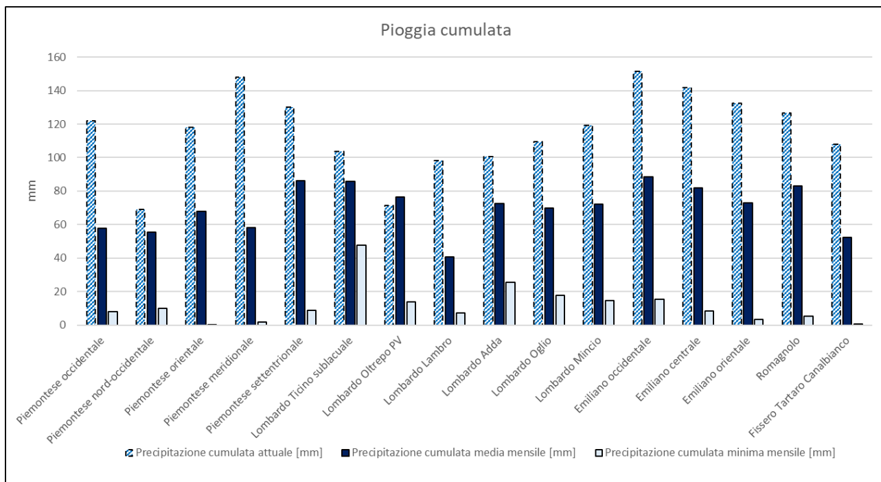
Figura 3: Confronto tra le precipitazioni attuali (al 31 marzo) e le precipitazioni cumulate storiche nelle aree idrografiche del Distretto.
