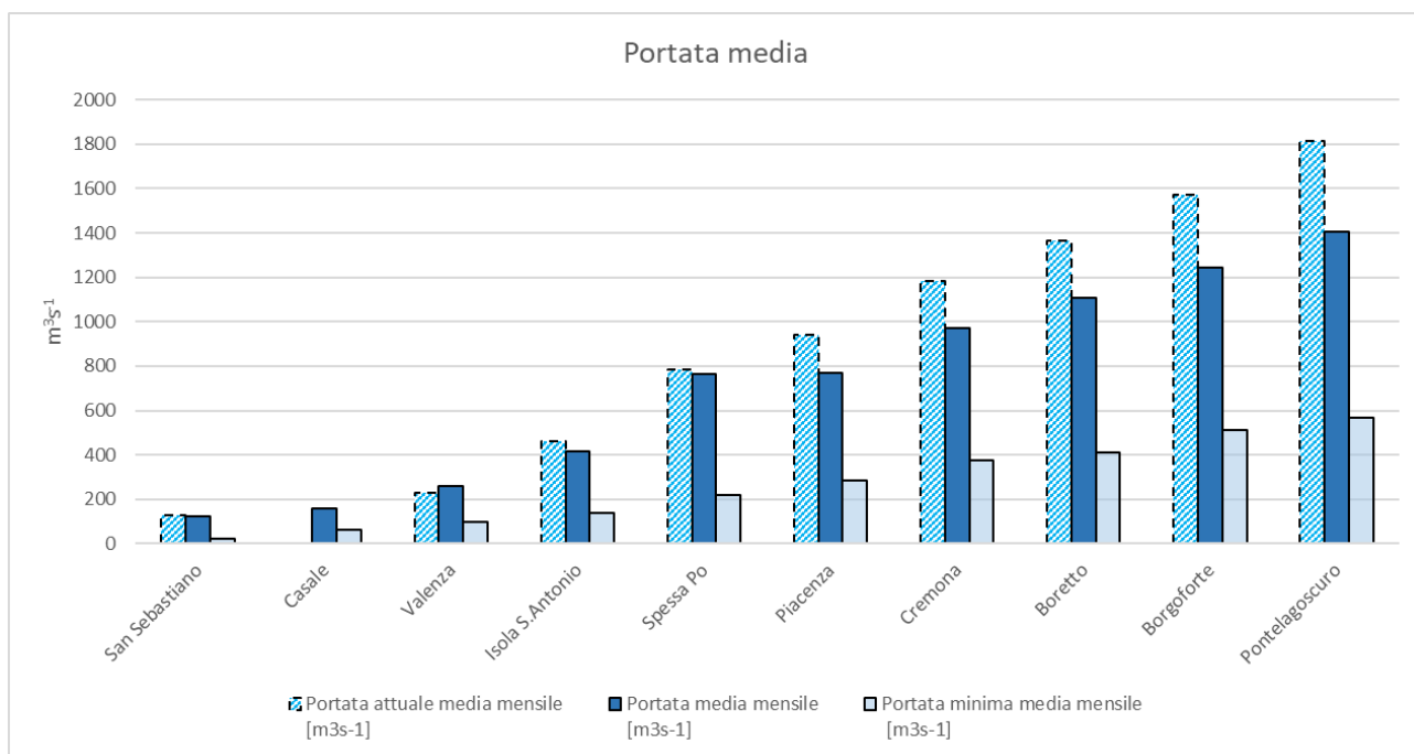
Figura 1: Confronto tra le portate medie attuali (marzo 2025) e le portate storiche del fiume Po.
