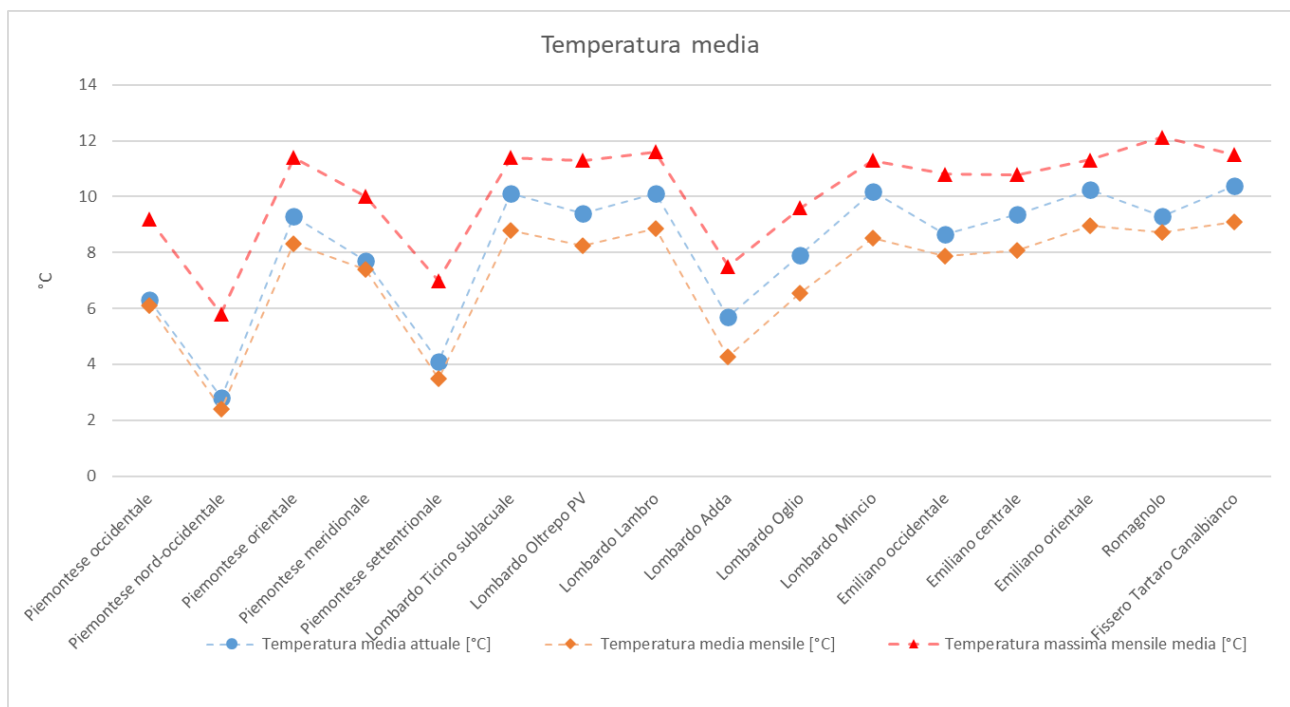
Figura 5: Confronto tra le temperature medie attuali (al 31 marzo) e le temperature di riferimento storiche, media e massima, nelle aree idrografiche del Distretto.
