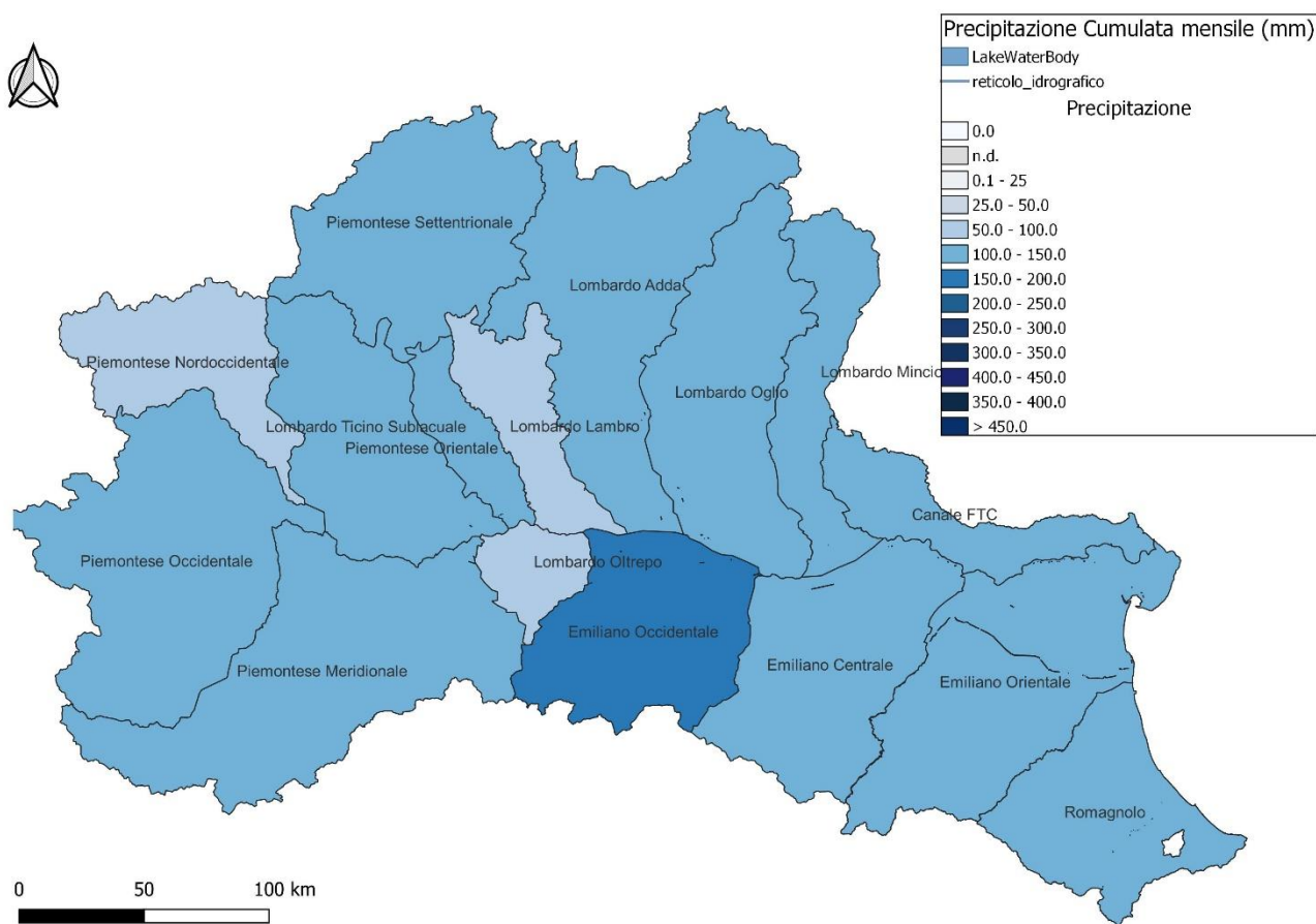
Figura 2: Rappresentazione della precipitazione cumulata nelle aree idrografiche del Distretto. Dati aggiornati al 31 marzo 2025.
